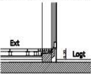
Schéma principe accès extérieur
