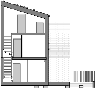
Coupe longitudinale
