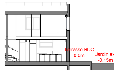
Coupe longitudinale
