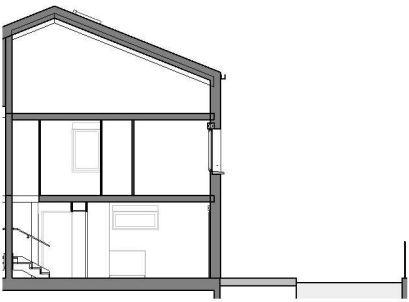
Coupe longitudinale
