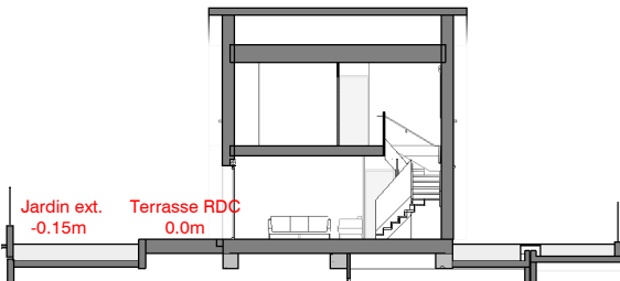
Coupe longitudinale
