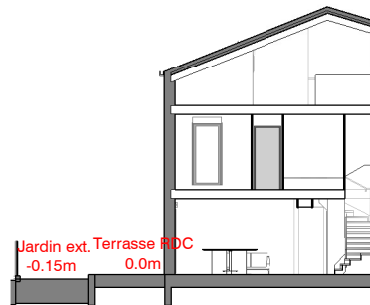
Coupe longitudinale
