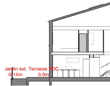
Coupe longitudinale
