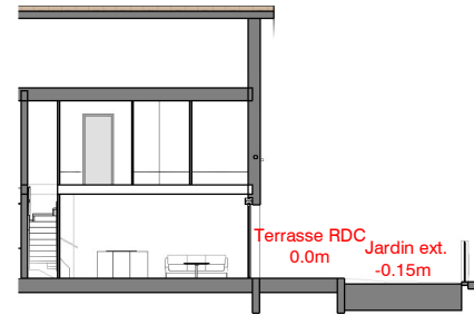
Coupe longitudinale
