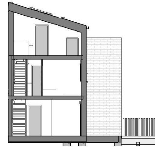
Coupe longitudinale
