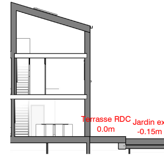
Coupe longitudinale
