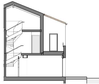
Coupe longitudinale
