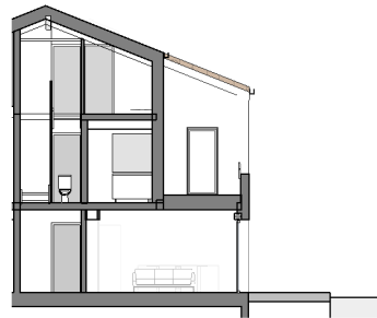
Coupe longitudinale
