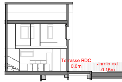
Coupe longitudinale
