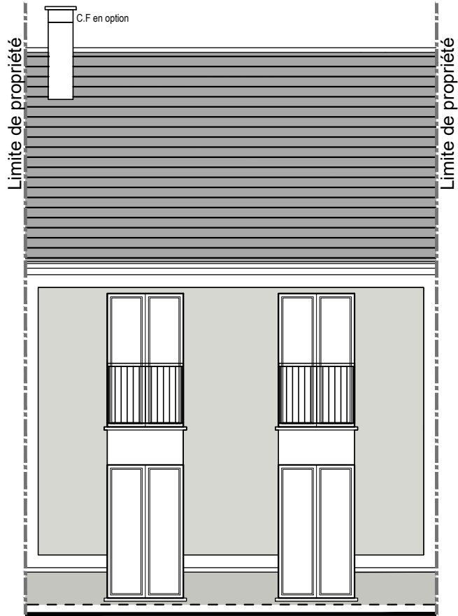
FACADE SUR JARDIN
