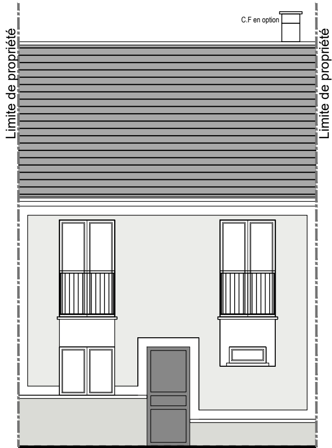
FACADE SUR ENTREE
