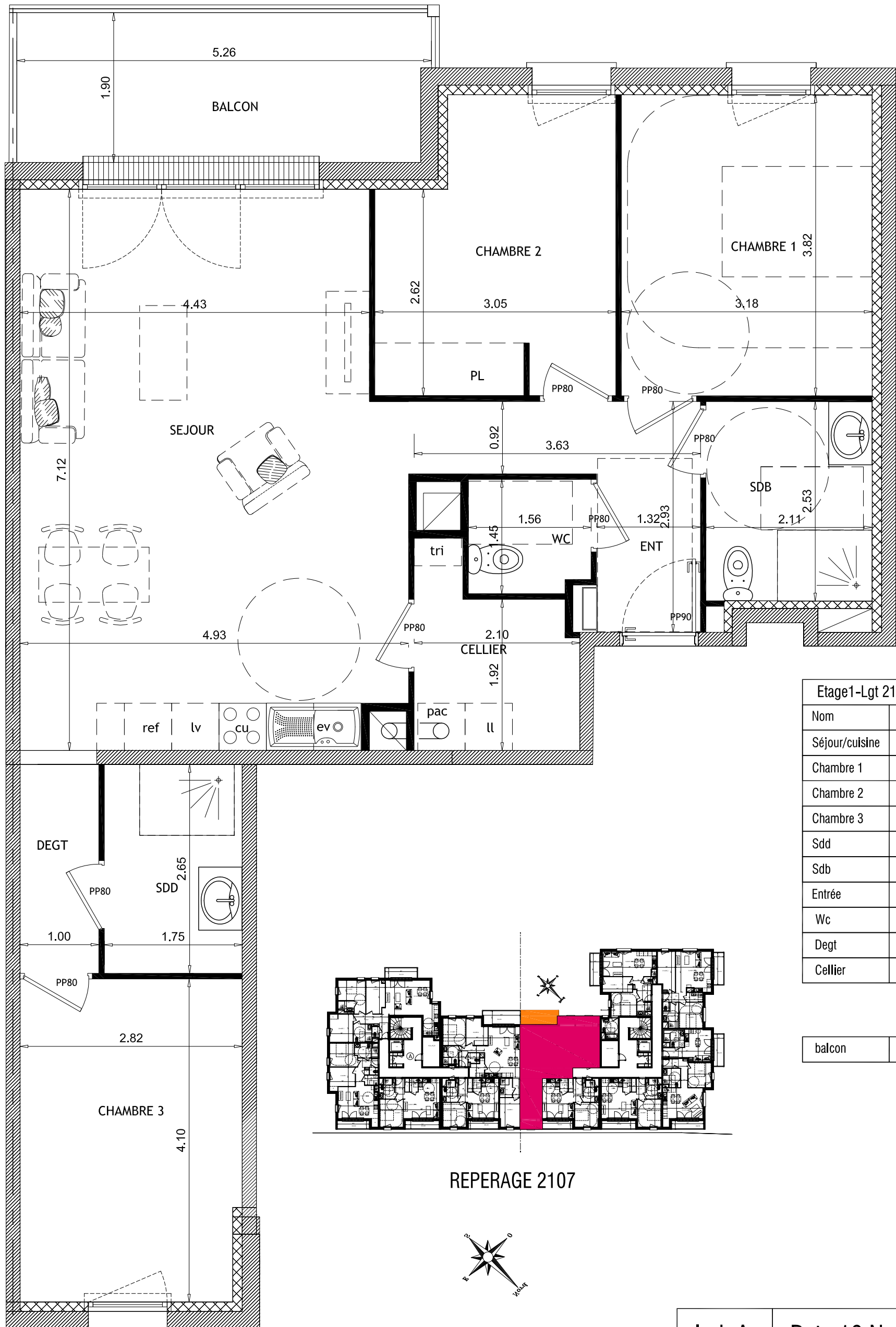
Plan de vente 2107 -ech 1/50eme
