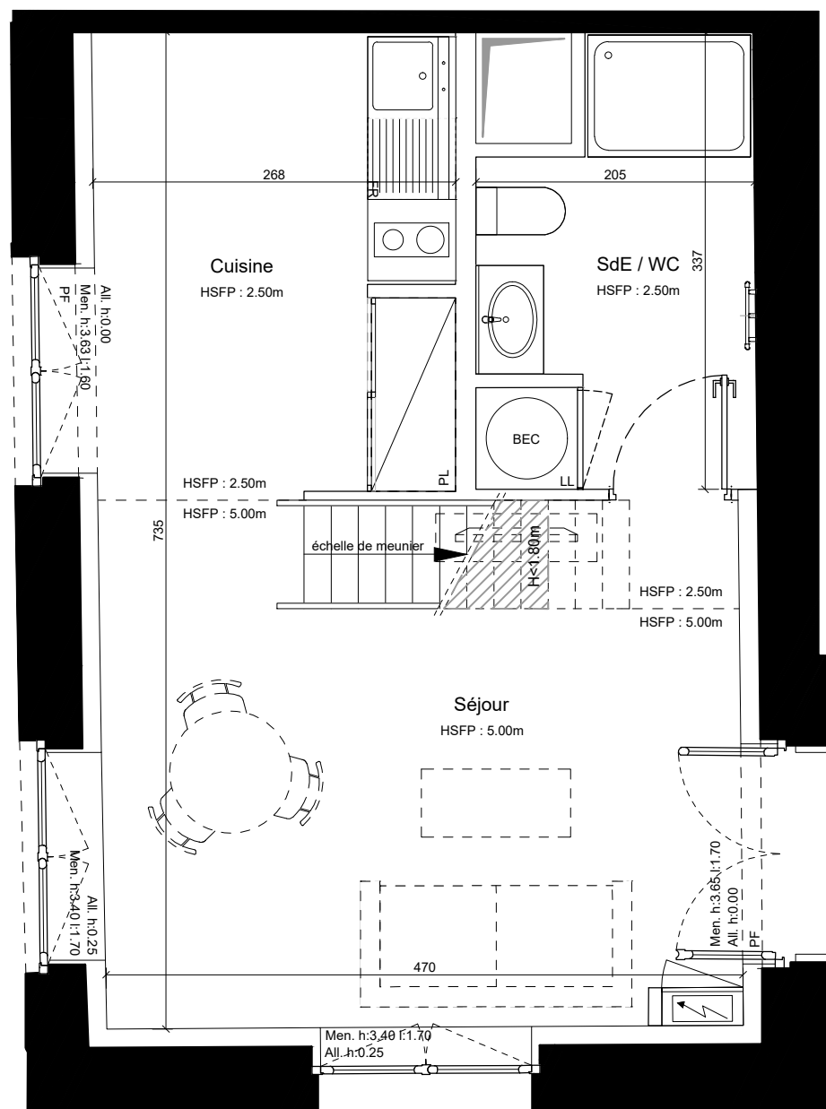
Plan RDC
