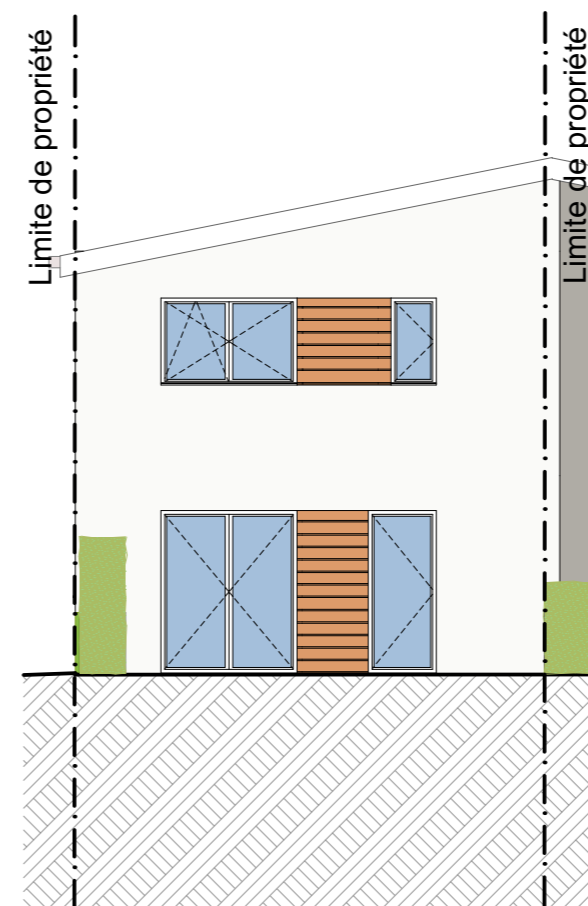
FACADE OUEST 1:100
