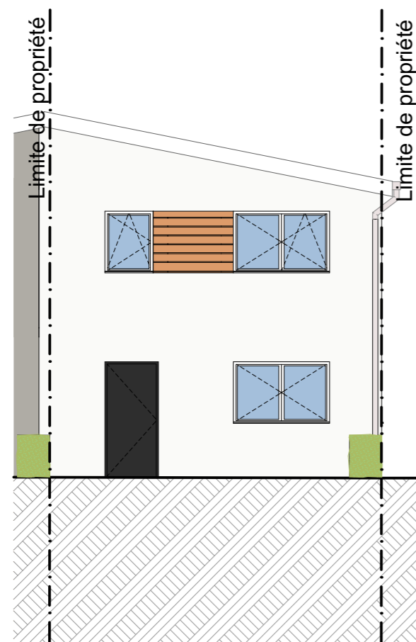
FACADE EST 1:100
