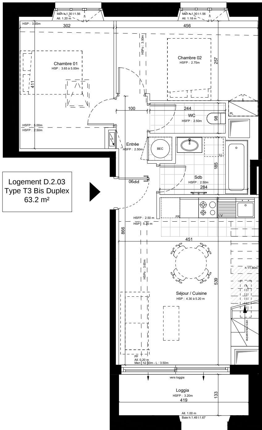
Plan R+2
