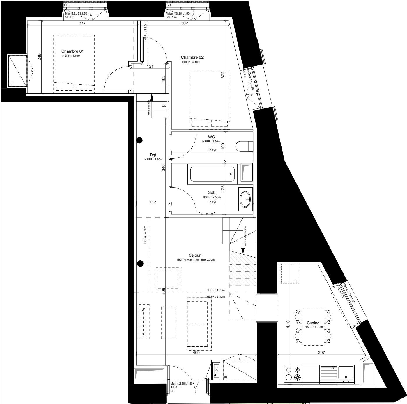
Plan RDC
